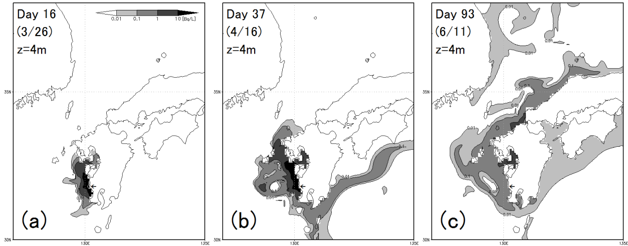
図1. 川内原子力発電所付近から流出したRIトレーサーの濃度分布
