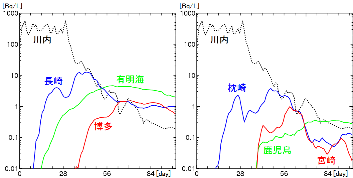
図2. 各沿岸海域におけるRI濃度の時間変化。横軸は3/11からの日数。
